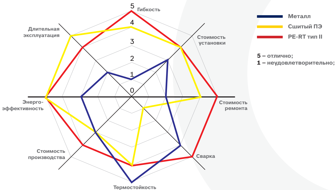
График 2. Эксплуатационные свойства различных материалов, применяемых во внутриквартирных трубопроводных системах
